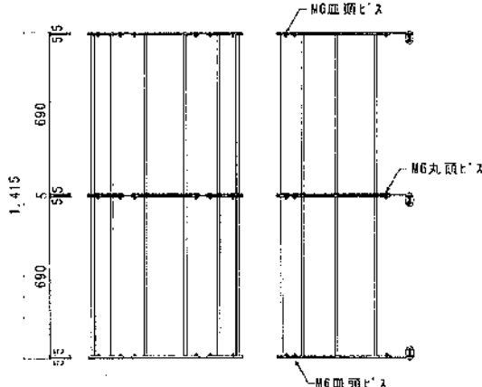
CAGE-14 ASタラップ用安全カゴ L=1,400
