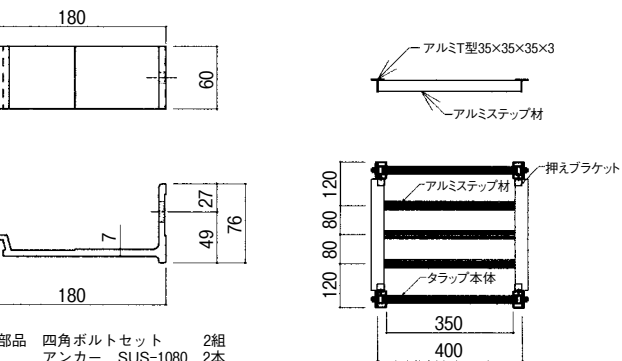
ブラケット BT-BK
