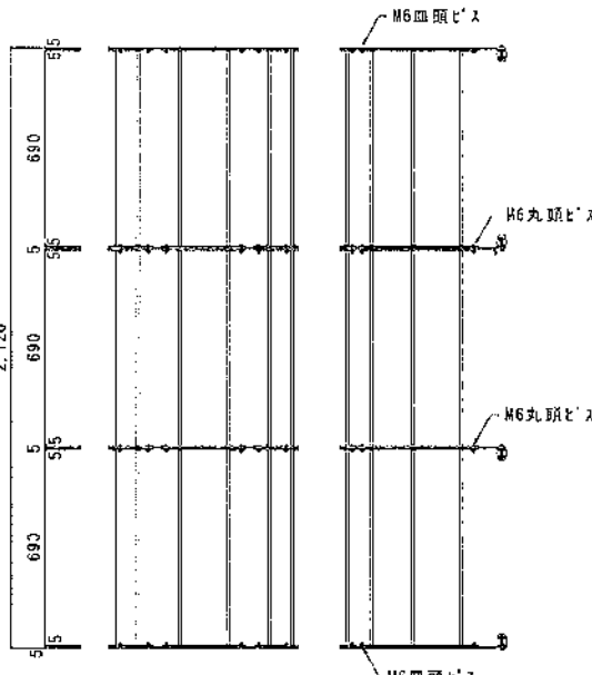
CAGE-21 ASタラップ用安全カゴ L=2,100
