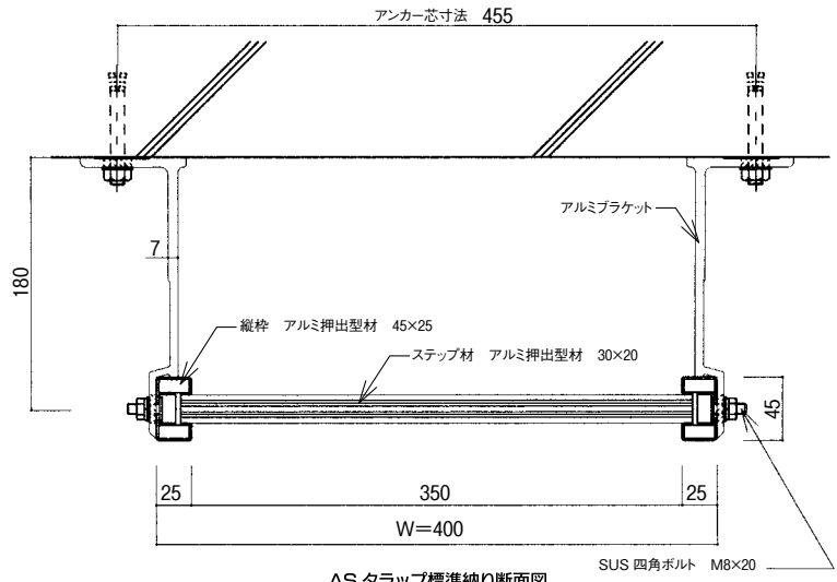
AS タラップ標準納り断面図
