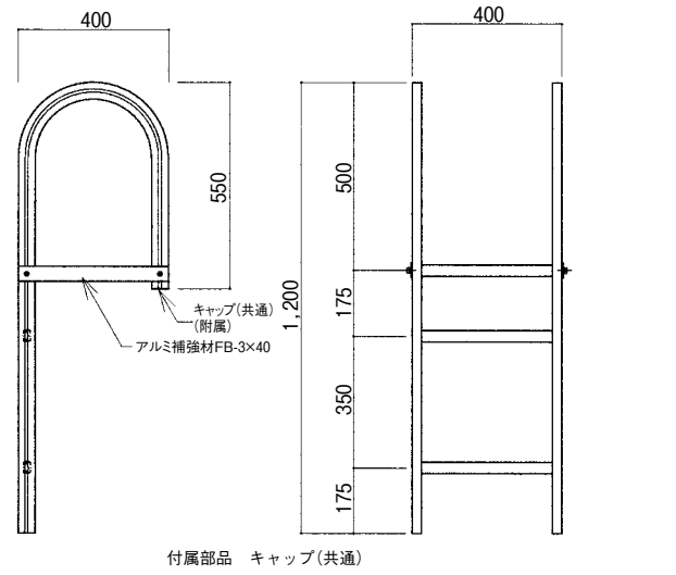
ASB-1 梯子頭部手掛
