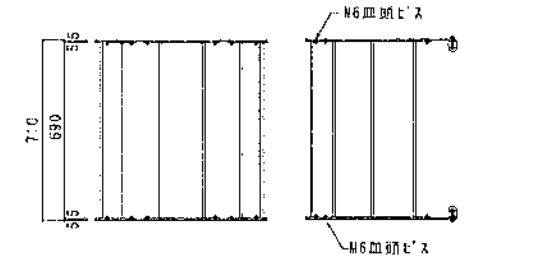
CAGE-07 ASタラップ用安全カゴ L=700
