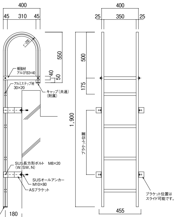
ASB-2姿図 S=1/10
